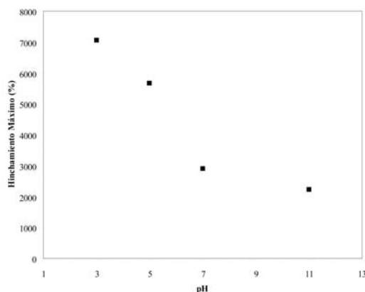
Fig. 3. Porcentaje de hinchamiento máximo como función del pH del medio de hinchamiento para los hidrogel de quitosana/FDS con una relación masa 5/1 y un porcentaje de sólidos totales del 4%.
