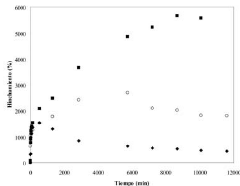
Fig. 4. Efecto del sobrehinchamiento para los hidrogel de quitosana/FDS con una relación masa 5/1 y un porcentaje de sólidos totales del 4% en diferentes medios de hinchamiento (■ pH 3, ○ pH 5 y ♦ pH 7).
